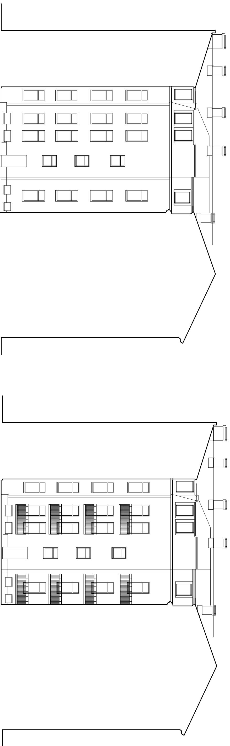
FASAD MOT GÅRD / SÖDER BEFINTLIGT UTSEENDE
