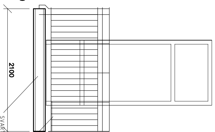
PRINCIP VV BALKONG 1:20
