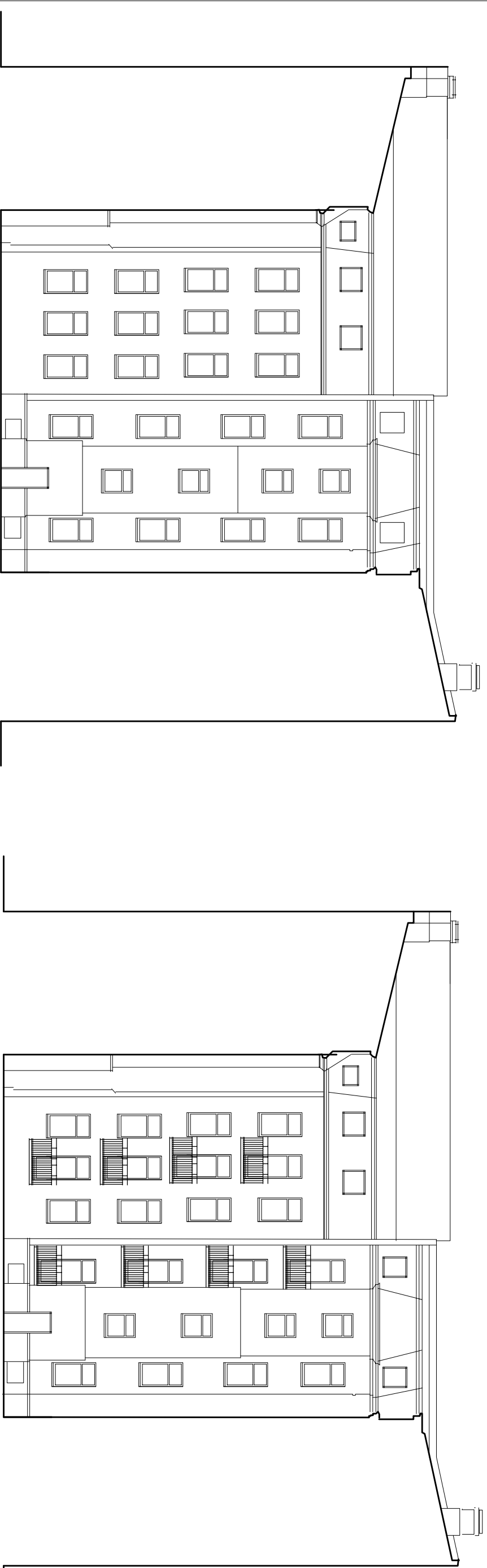
FAŠAD MOT GÅRD / ÖSTER BEFINTLIGT UTSEENDE
